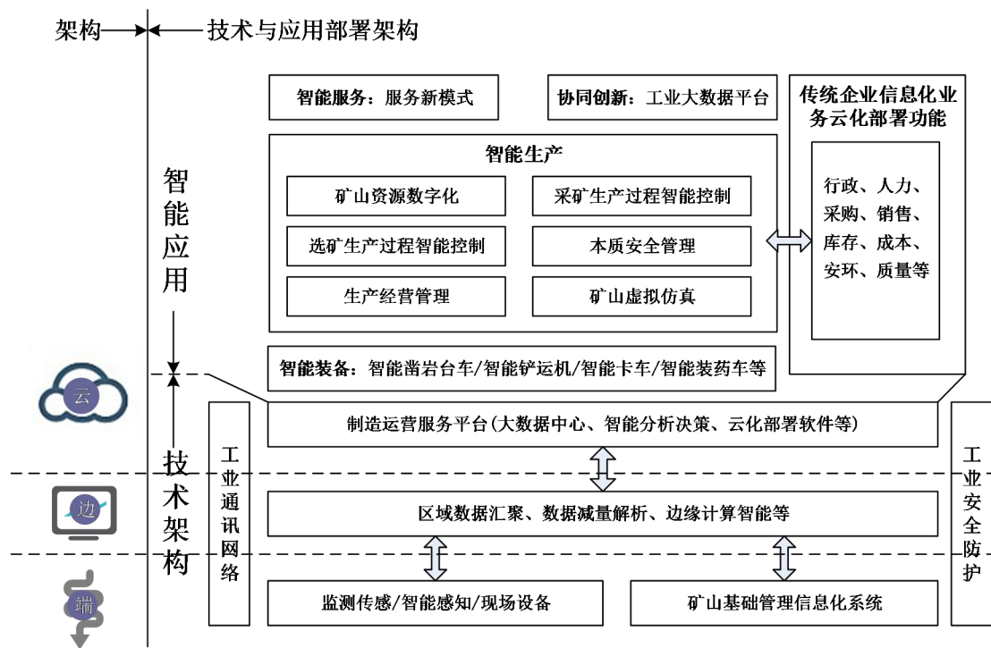
图 1 智能矿山总体架构图
